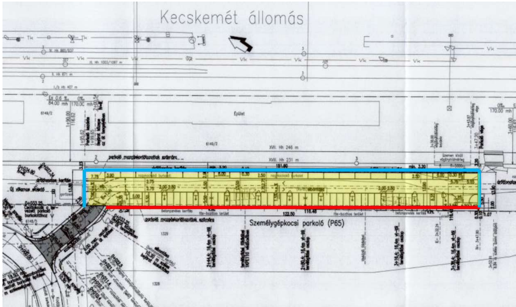
Részlet: Tervszám: 521/2017/1, Tárgy: Kecskemét vasútállomáson parkolók és útlehajtó létesítése, Rajzszám:P.01., 2018.03.09, Útépítés – Átnézeti helyszínrajz
