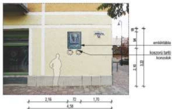
EMLÉKTÁBLA ELHELYEZÉSI TERV, M=1:50
