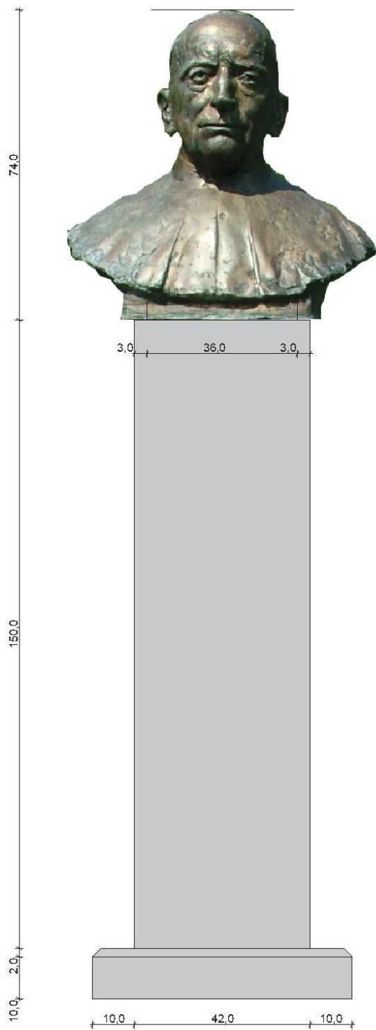
ELŐLNÉZET M=1:10
