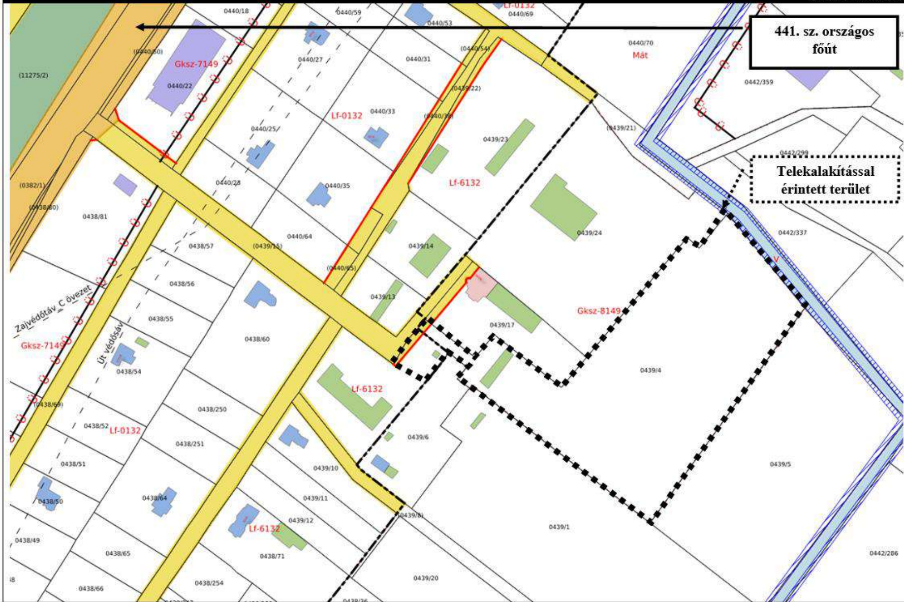
kivonat a hatályos szabályozási terv 25. sz. szelvényéből
