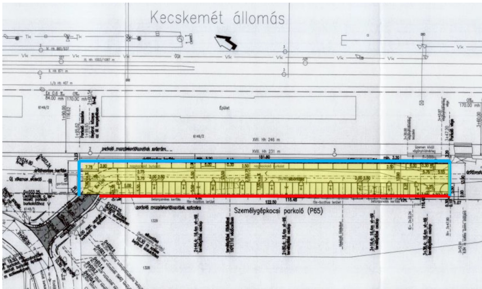
Részlet: Tervszám: 521/2017/1, Tárgy: Kecskemét vasútállomáson parkolók és útlehajtó létesítése, Rajkszám:P.01., 2018.03.09, Útépítés – Átnézeti helyszínrajz
