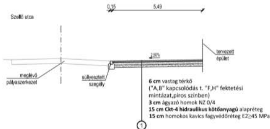
tervezett mintakeresztmetszervény
