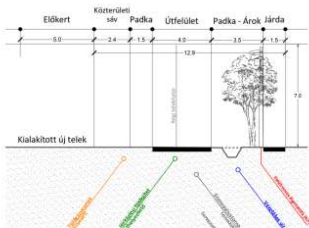
Javasolt keresztmetszvény
