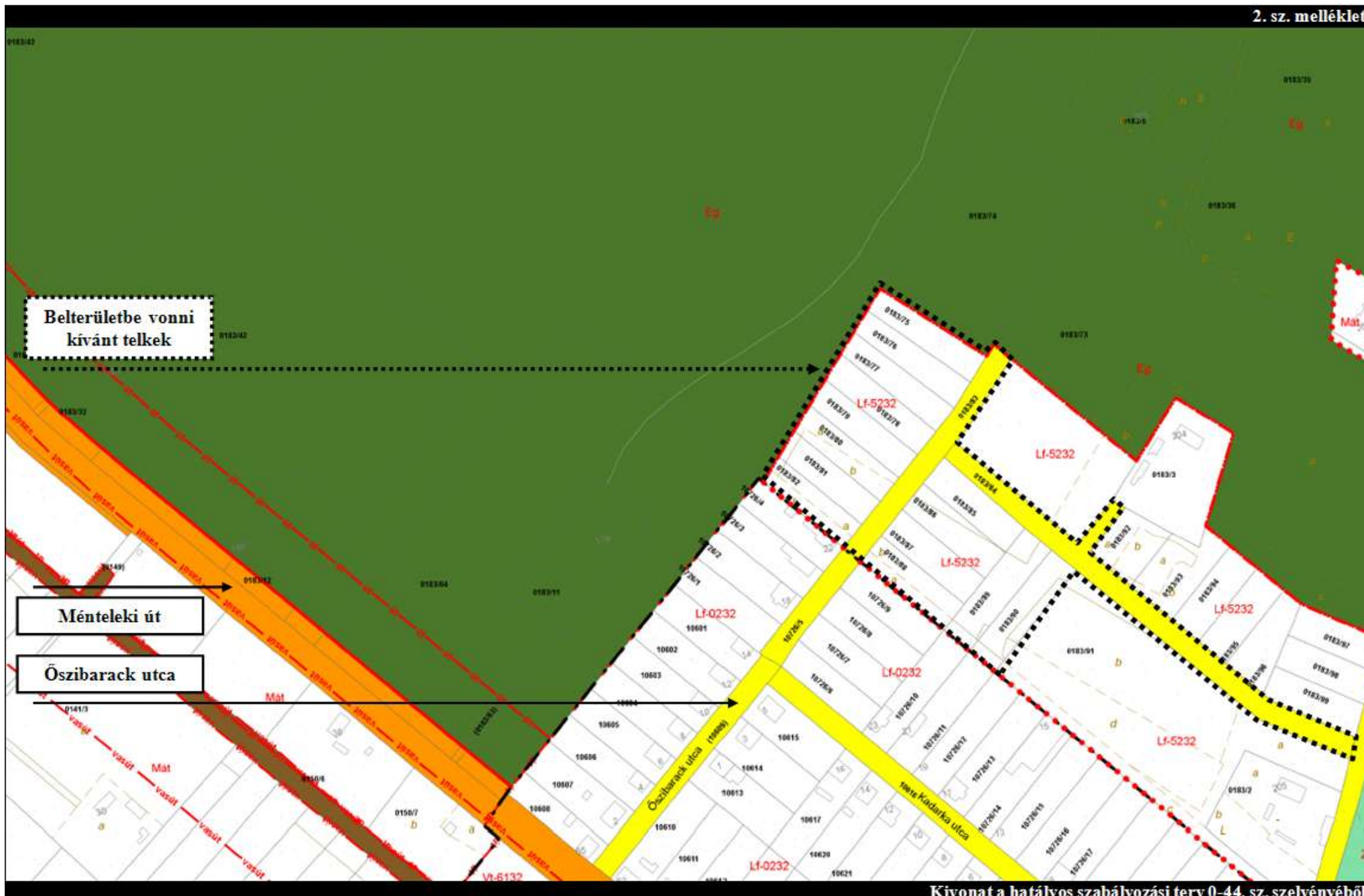
Kivonat a hatályos szabályozási terv 0-44. sz. szelvényéből
