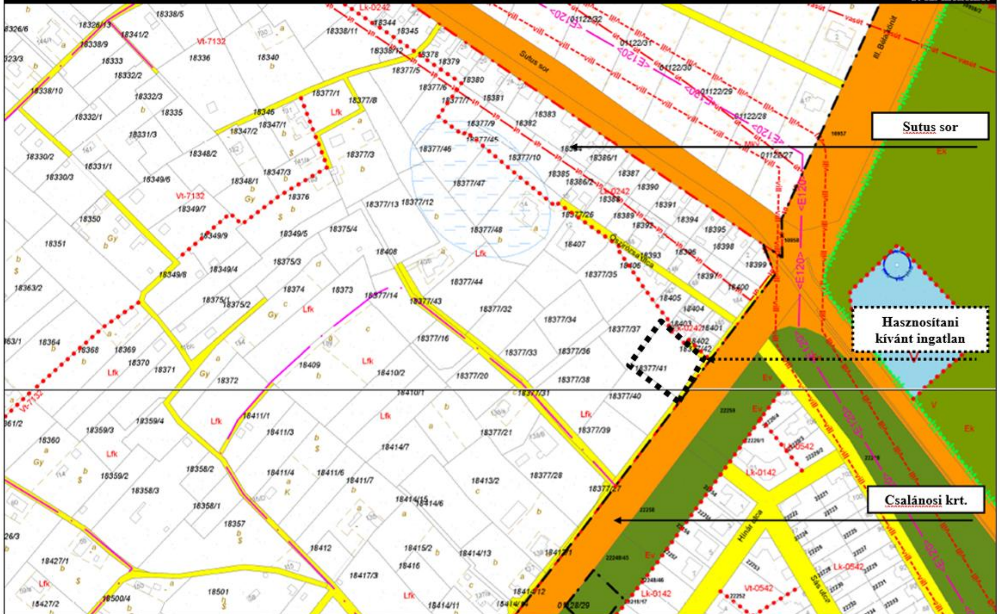
Kivonat a hatályos szabályozási terv 38-22 és 38-24. sz. szelvényekből
