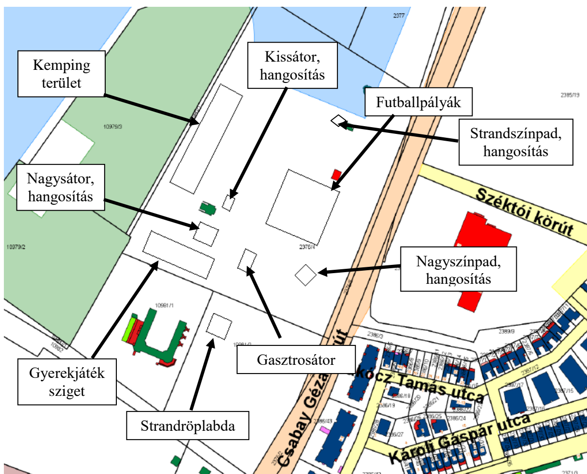
2. számú helyszínrajz
